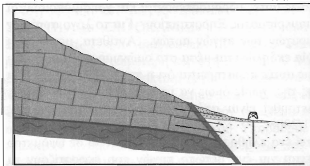
Εικόνα 2: Σχηματική γεωλογική τομή που απεικονίζει την υδραυλική επικοινωνία των καρστικών υδροφόρων οριζόντων με αυτούς που αναπτύσσονται μέσα στους μεταλλικούς σχηματισμούς.
